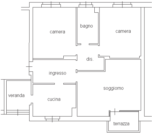
SECONDO PIANO H= 2,77
